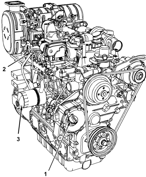
Рисунок 4 Двигатель C3.8 g02629297 (1) Крышка маслоналивной горловины (2) Масляный щуп (3) Масляный фильтр
